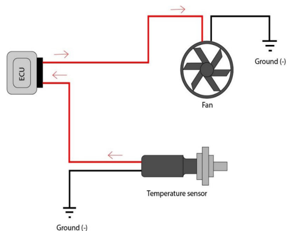
Foto 2. Esquema de principio de funcionamiento básico del ventilador controlado por ECU. Las flechas rojas marcan el flujo de información como corriente eléctrica
